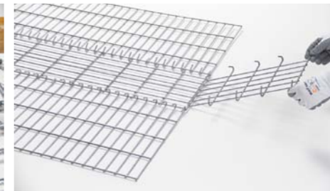
Sollevarre i laterali corti e avvicinarli per bloccarli con i laterali lunghi. Soulevez les côtés courts en les rapprochant du centre pour verrouiller avec les côtés longs.
